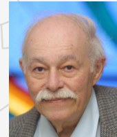
Abraham Lempel
